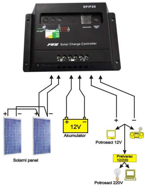
Šema veze regulatora sa panelima, akumulatorom i potrošačima
